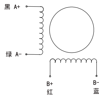
绕组接线图
